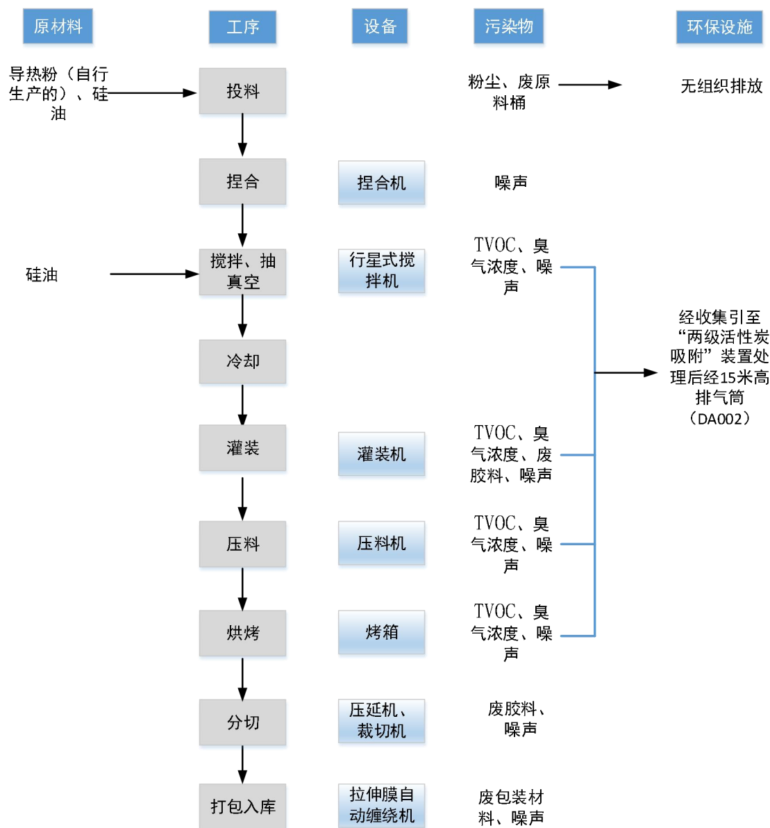
图 2-5 LED 封装胶生产工艺流程图
