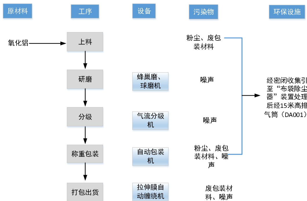
图 2-3 氧化铝生产工艺流程图
