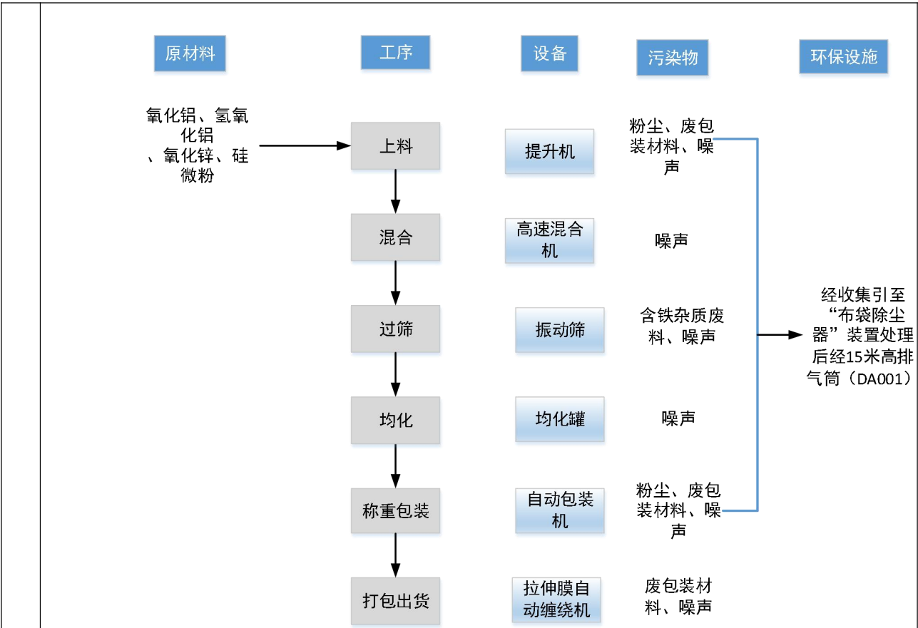
图 2-2 项目导热粉生产工艺流程及产污环节
